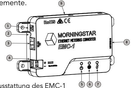
Abbildung 1-1. Ausstattung des EMC-1
