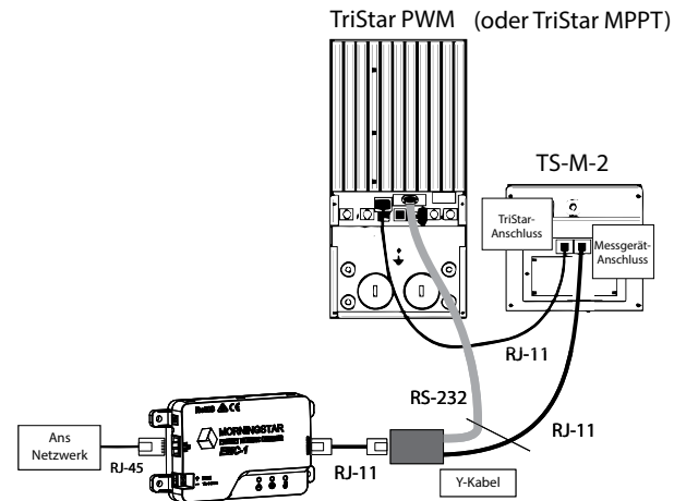
Abbildung 2-2. Anschluss von EMC-1 an TS-M-22. EMC
