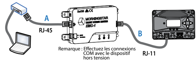
Figure 2-1. Connexion des câbles COM
