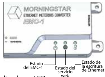
Figura 3-1. Indicadores LED
